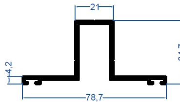
E-1712 0,786 kg/m
