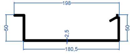
E-1401 2,108 kg/m
