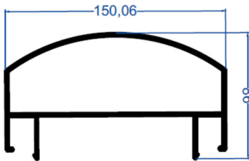
E-1341 2,298 kg/m
