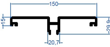
E-1706 1,535 kg/m
