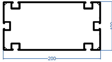
E-1710 4,734 kg/m
