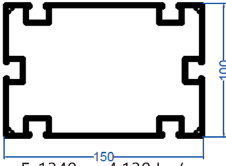
E-1340 4,130 kg/m
