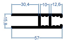
E-1707 0,760 kg/m
