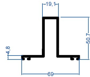
E-1624 0,824 kg/m
