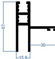
E-1711 0,931 kg/m
