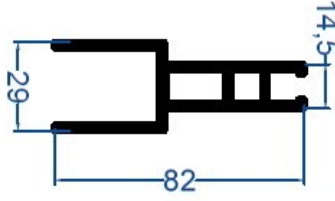
E-1708 1,093 kg/m
