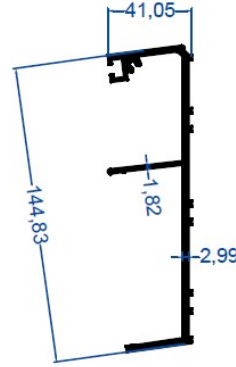
E-1847 2,068 kg/m Duvar Bağlantı ve "E" Kasa Profili
