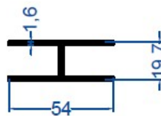
E-1843 0,558 kg/m "H" Profili
