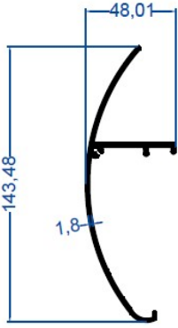
E-1846 1,126 kg/m Dere Kapak Profili
