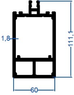
E-1840 2,306 kg/m Destekli Orta Kayıt Profili
