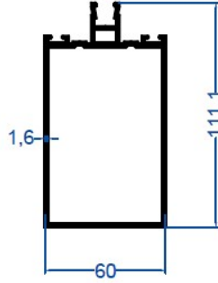
E1840/1 2,174 kg/m Orta Kayıt Profili
