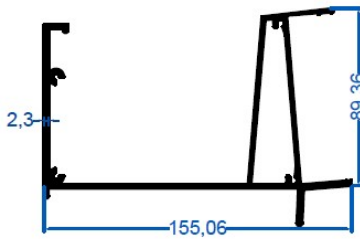
E-1848 3,008 kg/m Veranda Dere Profili
