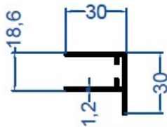
E-1844 0,312 kg/m "F" Profili
