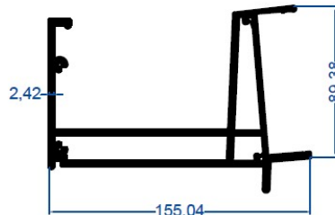
E-1839 3,837 kg/m Veranda Destekli Dere Profili
