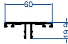
E-1849 0,476 kg/m Baskı Kapak Profili
