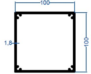
E-1045 2,135 kg/m 100 x 100 Kutu Profili
