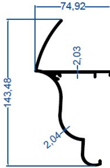
E-1845 1,472 kg/m Figürlü Dere Kapak Profili
