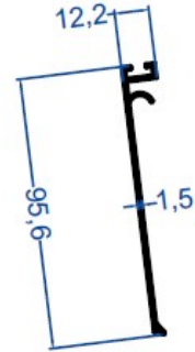
E-2130 0,510 kg/m Ön ve Arka Kapama Profili
