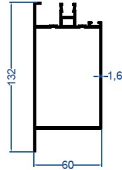
E-1851 1,778 kg/m Yan ve Köşe Kayıt Profili
