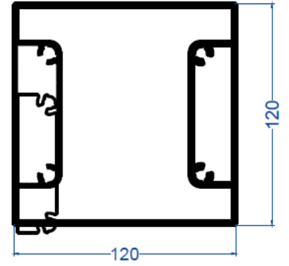
E-1262 4,264 kg/m Ayak Profili
