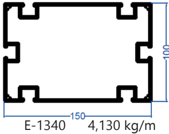
E-1340 4,130 kg/m Taşıyıcı Kutu Profili 100x150
