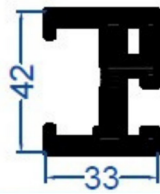
E-12395 1,626 kg/m Üst Ray Profili
