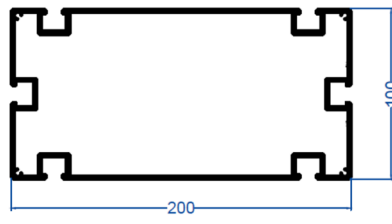
E-1710 4,734 kg/m Taşıyıcı Kutu Profili 100x200
