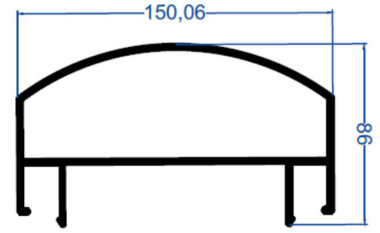
E-1341 2,298 kg/m Su İnış ve Tahliye Profili
