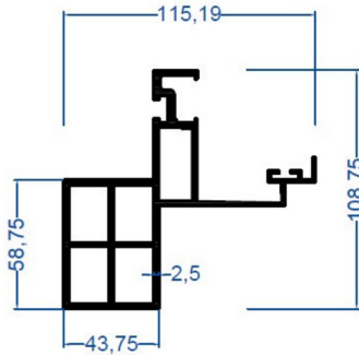
E-12394 8,300 kg/m Ana Ray ve Yan Dere Profili
