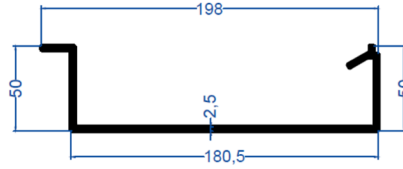
E-1401 2,108 kg/m Dere Alt Profili
